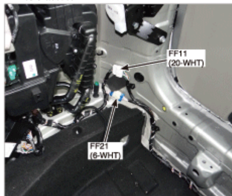
115.行李箱后右
