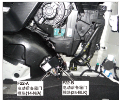
117.行李箱右侧
